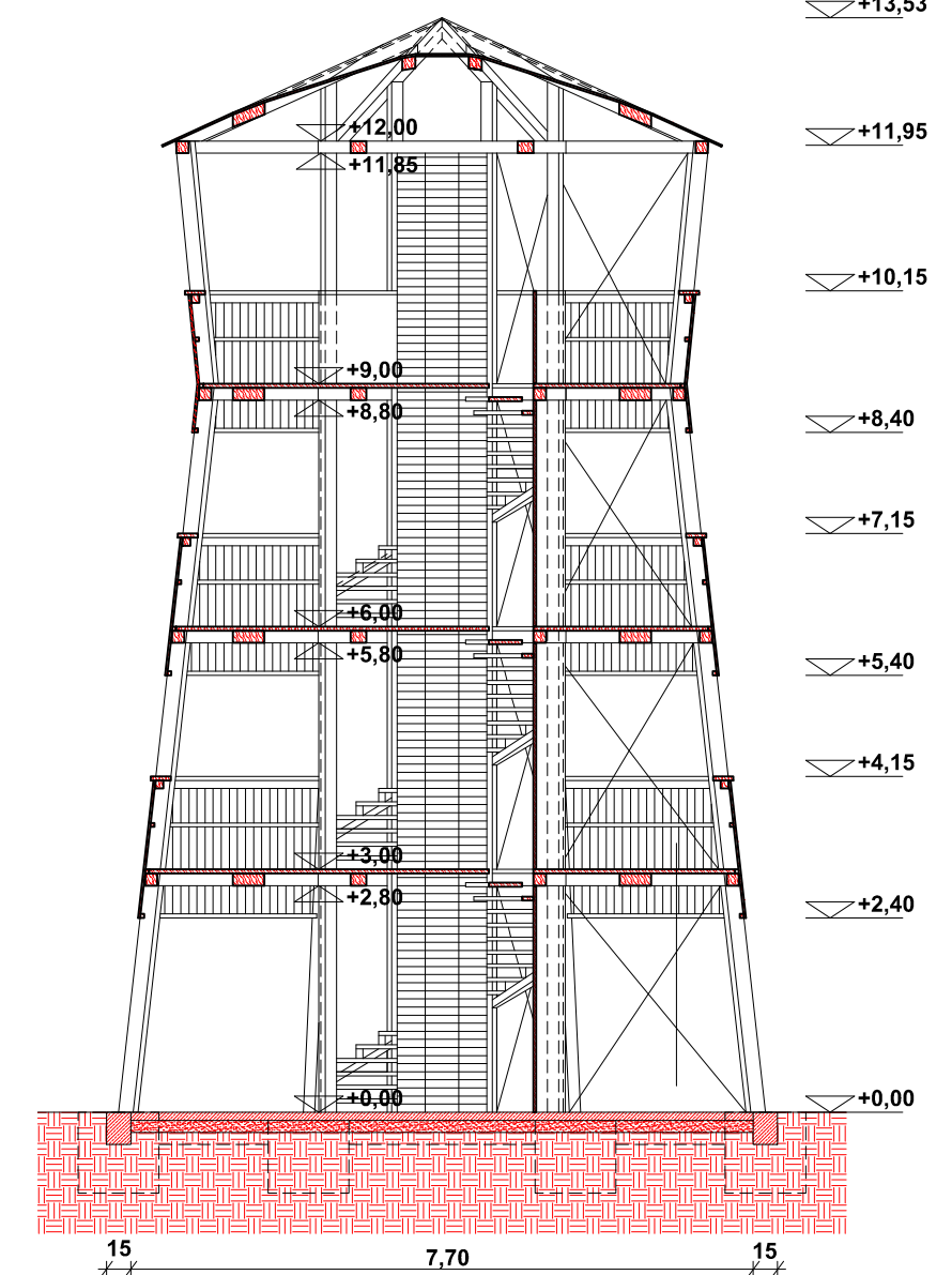
A-A METSZET
